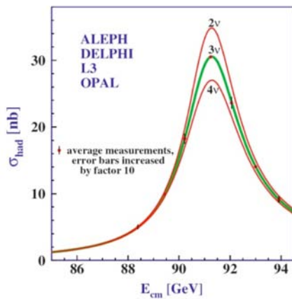
Figura 1: Misure a LEP della larghezza di decadimento del bosone Z^0 . I punti sperimentali sono confrontati con differenti modelli che prevedono 2, 3 o 4 famiglie di neutrini. Come si osserva facilmente, i dati sperimentali suggeriscono l'esistenza di sole 3 famiglie neutriniche (curva verde). Si noti che gli errori sperimentali sono stati ingranditi 10 volte per renderli visibili, quindi l'accordo col modello a 3 neutrini è molto forte.
